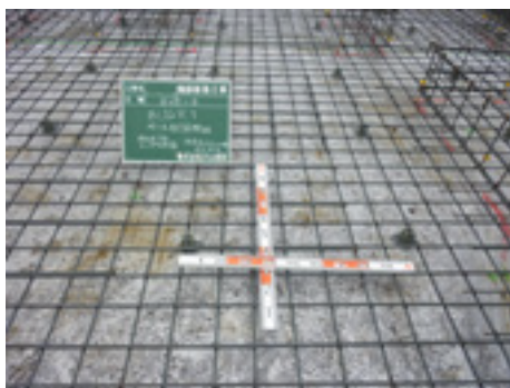
べた基礎の鉄筋工事
